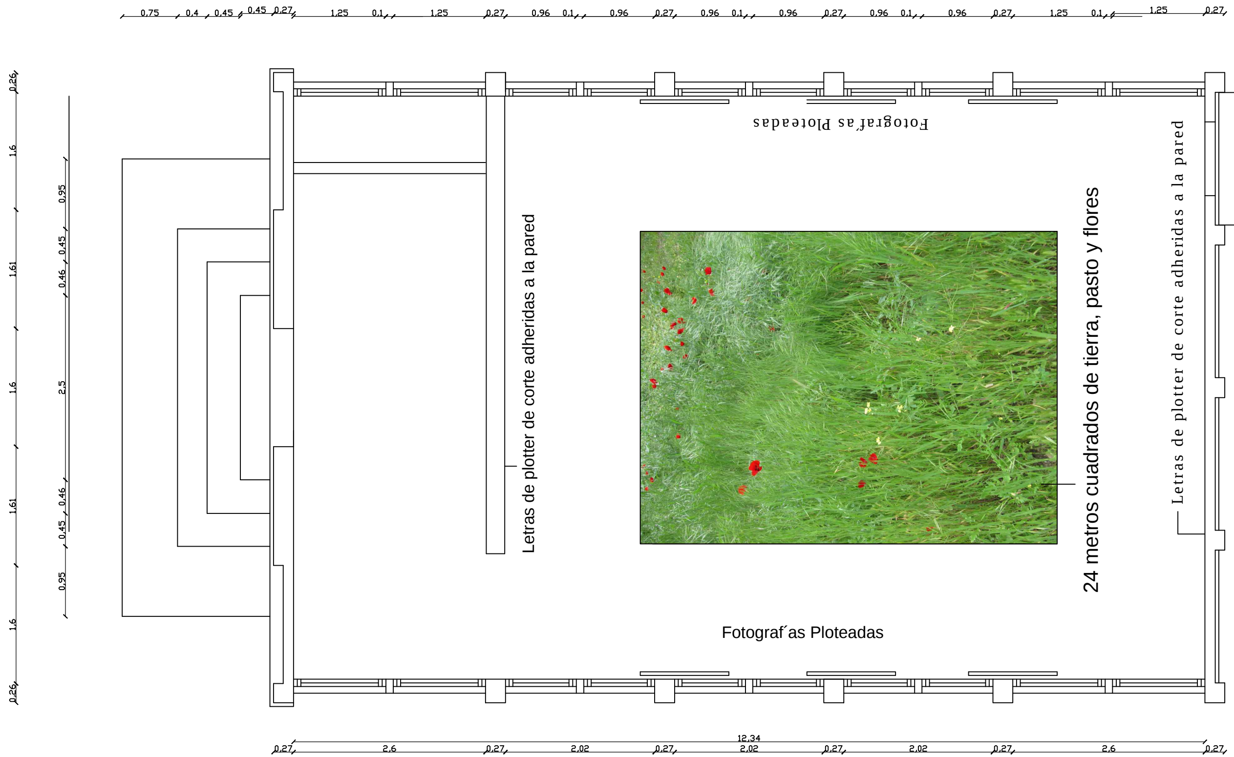
Planta esc 1: 50
