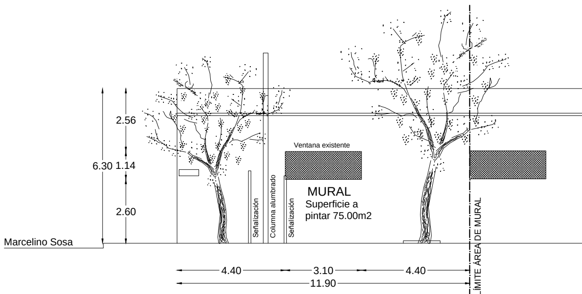
FACHADA C. REYLES ESC. 1:150
