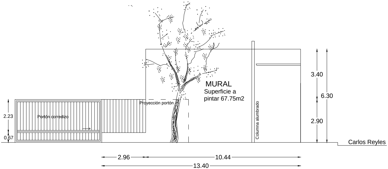
FACHADA M. SOSA ESC. 1:150
